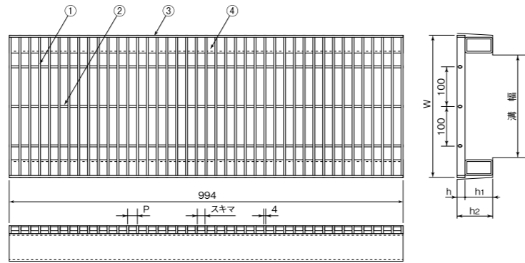
部品構成 材質:SUS304 ①メインバー ②クロスパイプ ③エンドバー ④かさ上げ材
